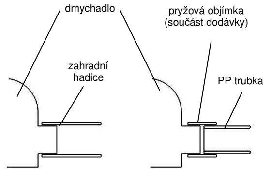
Připojení přívodu vzduchu do nádrže k dmyhadlu
