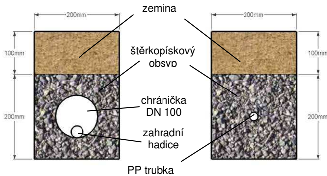
Uložení přívodu vzduchu do nádrže
