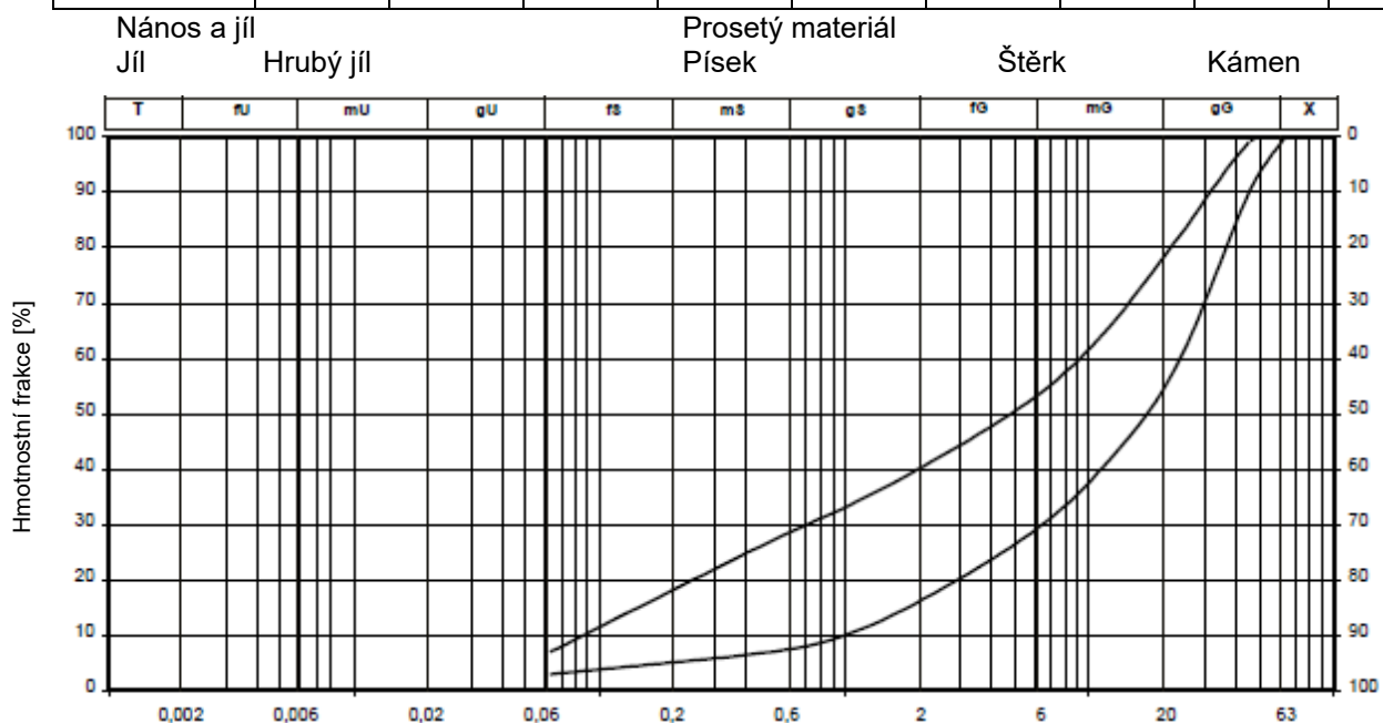
Obrázek č. 8: Křivka zrnitost 0/45 (směs by se měla nacházet v dolní části křivky doporučené rozmezí zrnitosti, avšak požadavky na funkčnost směsi mají v takovém případě přednost) Průměr zrna [mm]
