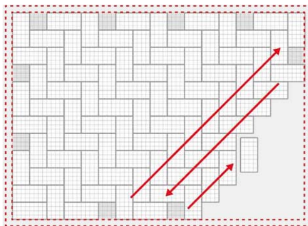
Obrázek č. 11: Navzájem se uzamykající prvky (vysoký/nizký obrubník) – v případě nezbytnosti zamčené hraniční desky
