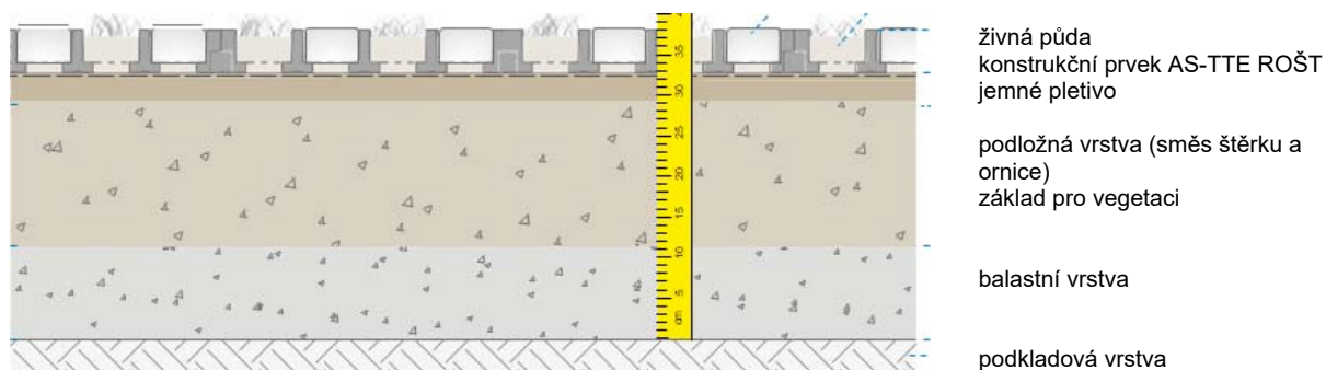
Obrázek č. 3: Zatravněný systém AS-TTE ROŠT konstrukční princip 3
