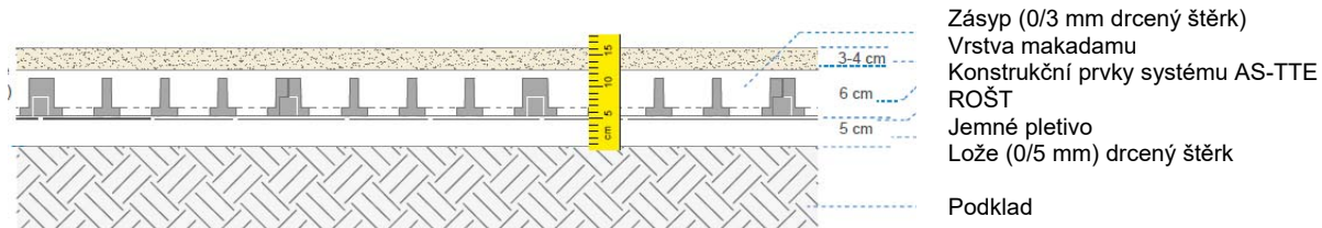
Tabulka č. 17: Systém AS-TTE ROŠT s povrchovou vrstvou (např. u Konstrukčního principu 1)
