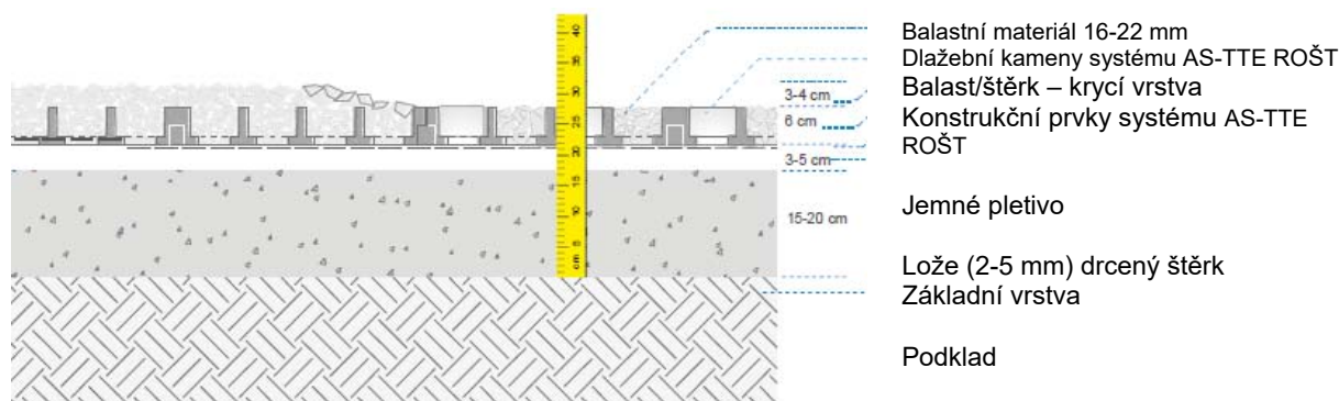
Tabulka č. 16: Systém AS-TTE ROŠT se štěrkovou povrchovou vrstvou (např. u Konstrukčního principu 2)
