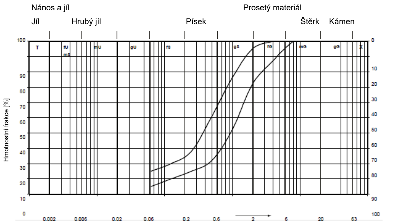
Obrázek č. 9: Doporučená křivka zrnitosti pro podkladové vrstvy vegetace (zásypového materiálu u zelených povrchů; směs by se měla nacházet v dolní části křivky doporučeného rozmiřnosti, avšak požadavky na funkčnost směsi mají v takovém případě přednost)
