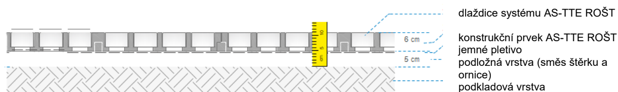
Obrázek č. 4: Zpevněný (dlážděný) systém AS-TTE ROŠT konstrukční princip 1
