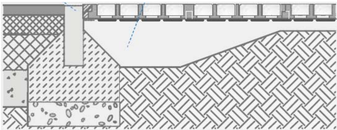
Obrázek č. 10: Konstrukční princip 1 systému AS-TTE ROŠT s klínovitě tvarovanou podkladní vrstvou pro zajištění lepšího zarovnání povrchu v hraničních oblastech, přes které se přejezdí.
