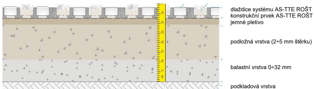
Obrázek č. 6: Zpevněný (dlážděný) systém AS-TTE ROŠT konstrukční princip 3
