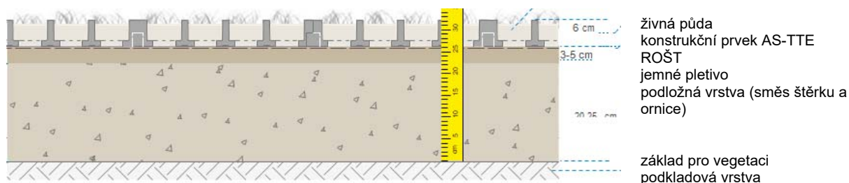
Obrázek č. 2: Zatravněný systém AS-TTE ROŠT konstrukční princip 2
