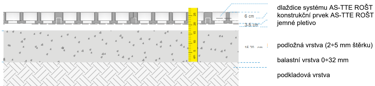
Obrázek č. 5: Zpevněný (dlážděný) systém AS-TTE ROŠT konstrukční princip 2
