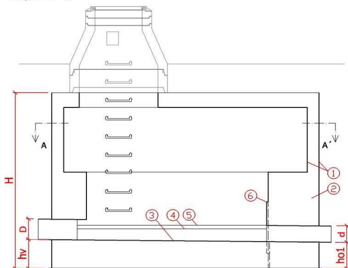
Řez B-B'
