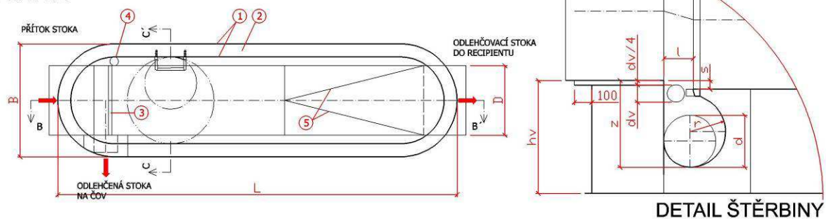
Řez A-A'
