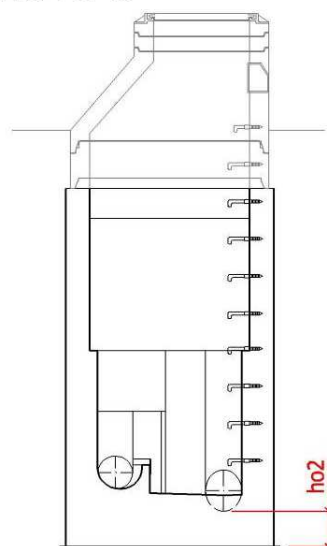
Řez C-C'
