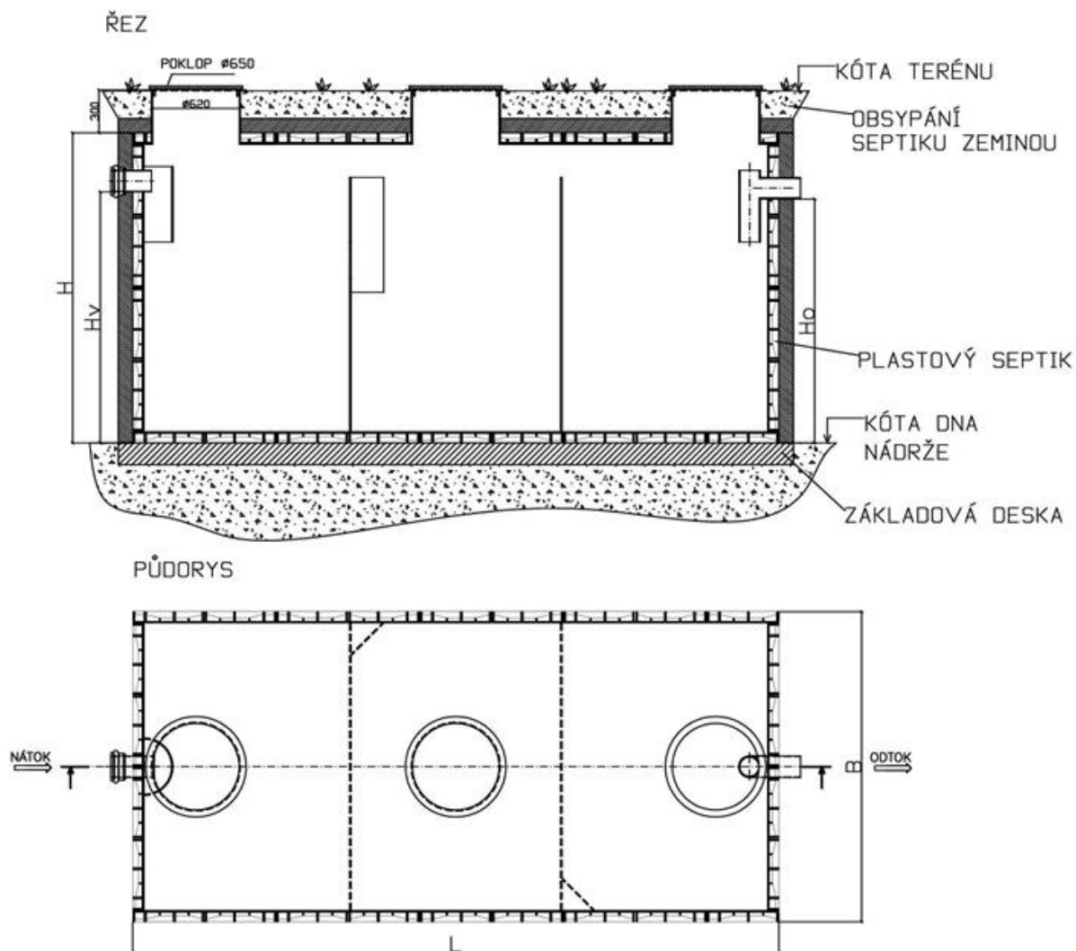
Obr. č. 2 - Rozměrové schéma typu PP septiků hranatých /ER/ -pro obetonování
